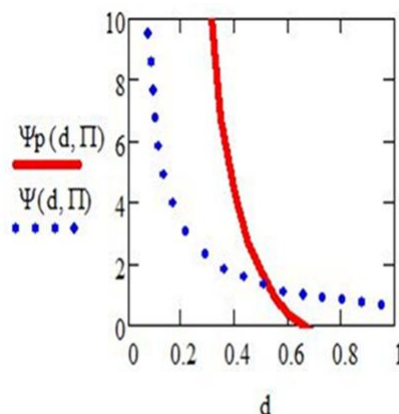
Рис. 2: Рост экономики при распределениях Туганова-Цея ( Y ) и Парето ( Y_p )
