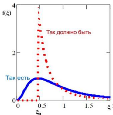
Рис. 1: Распределения Парето и Туганова-Цея
